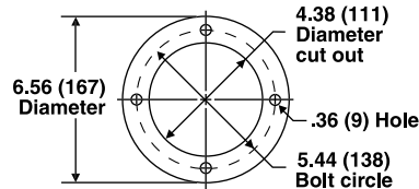
VERSA FLANGE BOLT CIRCLE
