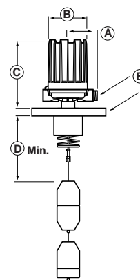
Séries B15 - Montage à bride
