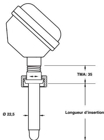
DIN 11851
