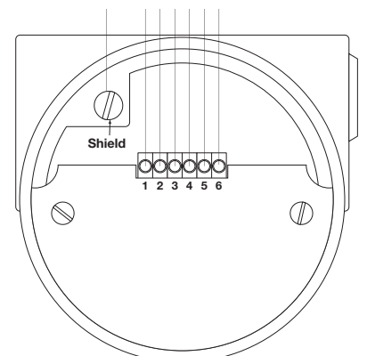
Connexions sonde TD2 électronique déportée
