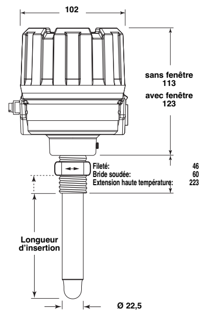
Modèle TD2 avec électronique intégrée et sonde à embout sphérique TMA/TMB
