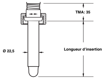
DIN 11851
