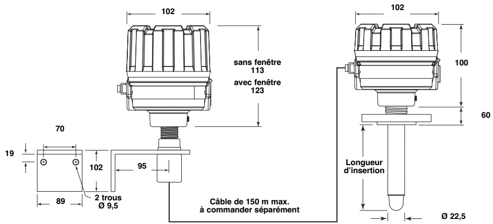
Modèle TD2 avec électronique déportée
