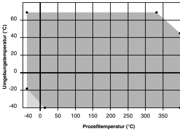
Zulässige Betriebsbedingungen Stahlgußgehäuse mit Silberkontakten mit Silber-/Goldkontakten HS
