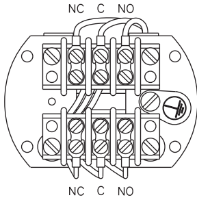
Klemmenanschluß DPDT Mikroschalter mit Silberkontakten
