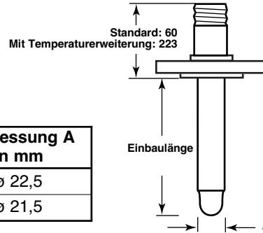
Sensor mit Flanschanschluss
