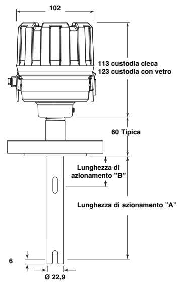
962 - Connessione flangiata
