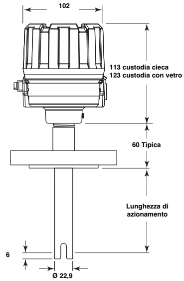
961 - Connessione flangiata
