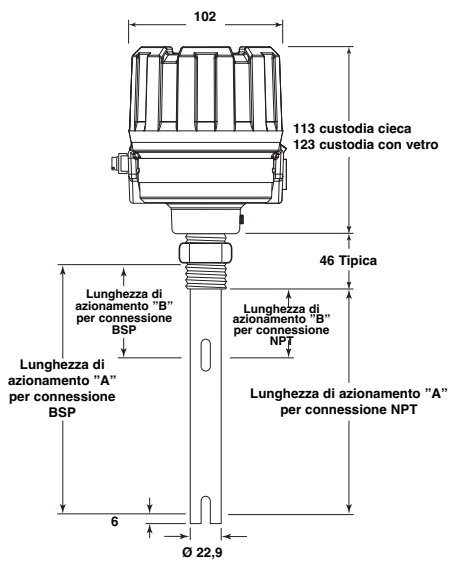
962 - Connessione filettata
