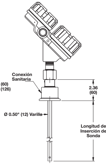
Eclipse® con Sonda 7xF-E Conexión Higiénico
