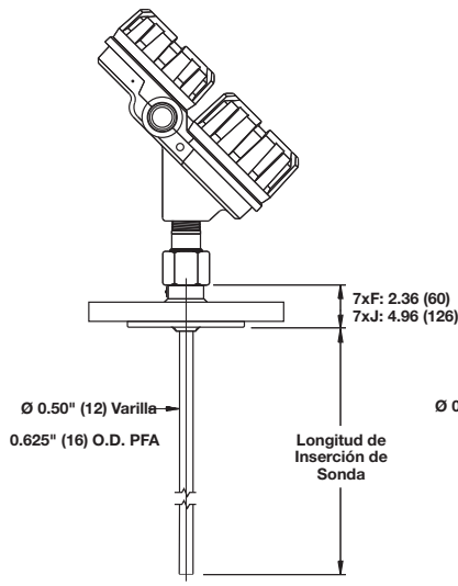
Eclipse® con Sonda 7xF de Conexión Bridada
