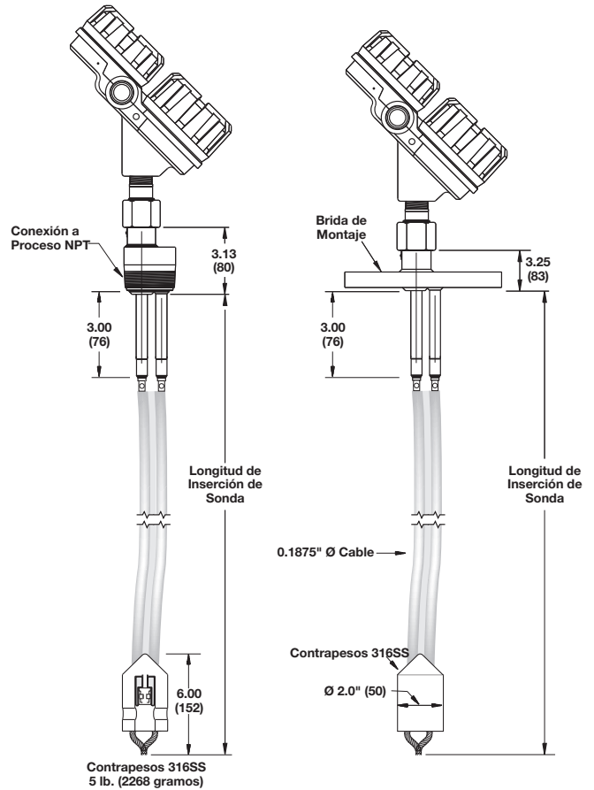
Eclipse® con Sonda de Varilla Gemela Flexible para Sólidos Gruesos 7x5, Conexión Bridada o NPT
