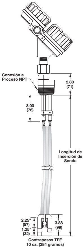
Eclipse® con Sonda de Varilla Gemela Flexible 7x7 Conexión Bridada o NPT
