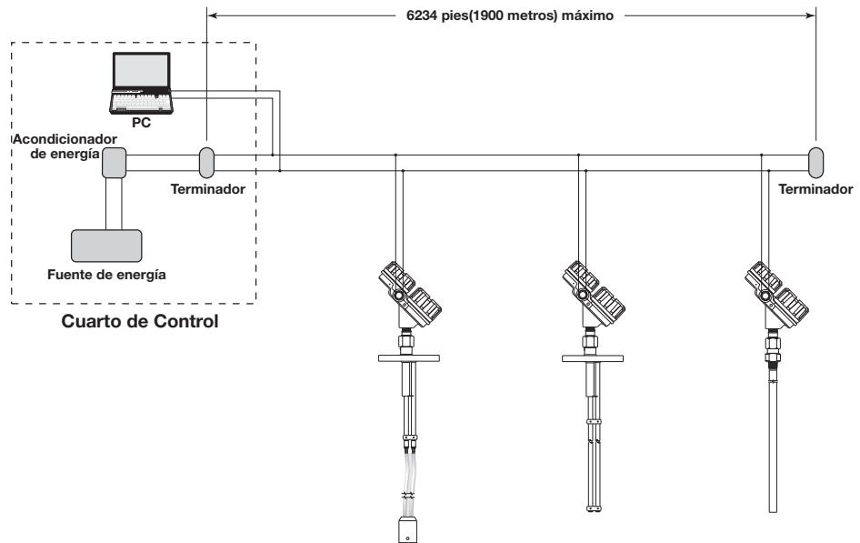
Instalación Fieldbus típica
