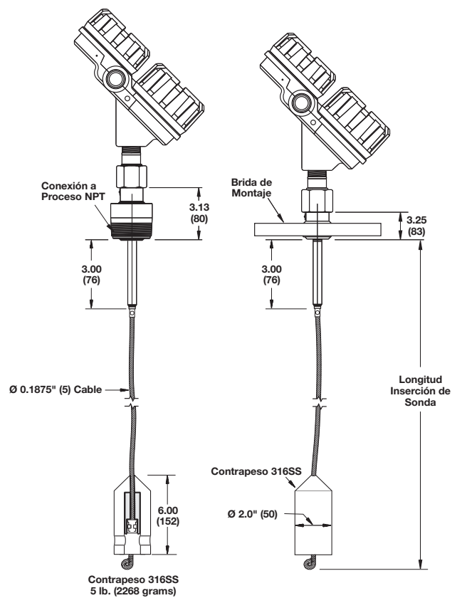
Eclipse® con Sonda Flexible para Sólidos Gruesos 7x2 Conexión Bridada o NPT
