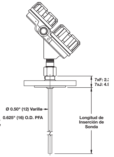
Eclipse® con sonda 7xF-F Conexión con Brida
