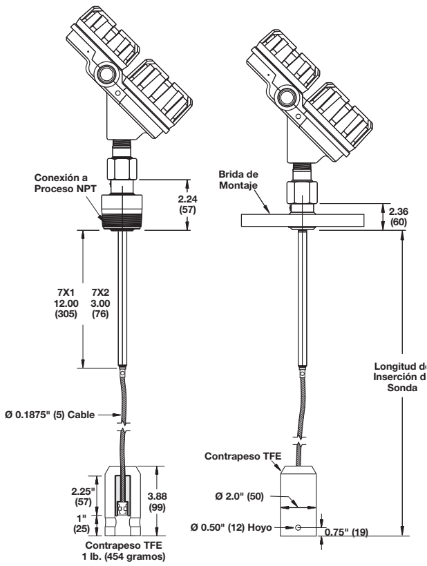
Eclipse® con sonda Flexible 7x1 Conexión Bridada o NPT
