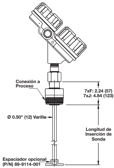
Eclipse® con Sonda 7xF de Conexión Roscada NPT
