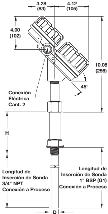
Eclipse® con sonda 7XS Conexión Roscada
