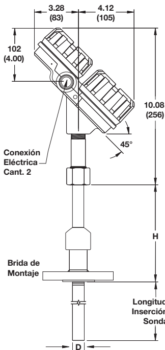
Eclipse® con sonda 7XS Conexión Bridada
